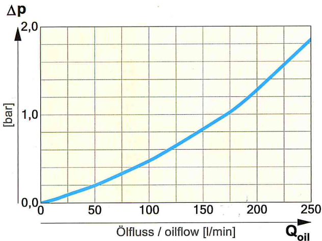
pressure drop at 30 cst Druckabfall bei 30 cst
