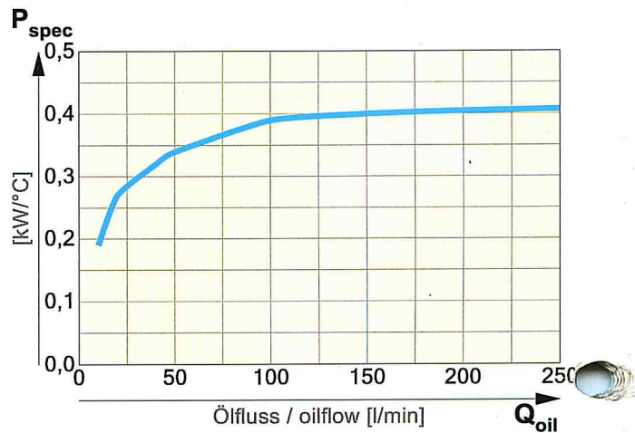
specific heat dissipation spezifische Kühlleistung
